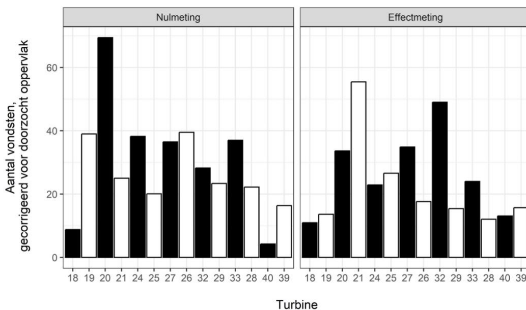
Figuur 3.2 Verdeling van de slachtoffers over de turbines in de nulmeting (links) en het eerste jaar effectmeting (rechts). De aantallen zijn gecorrigeerd voor het doorzocht oppervlak, maar niet voor vindkans en verdwijnsnelheid. De zwarte en witte staven geven respectievelijk de impact- en controleturbines weer. Dit is van links naar rechts per setje weergegeven (18 en 19, 20 en 21 enz.).
