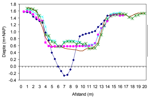
Doorstroomprofiel kreek locatie 6-6
