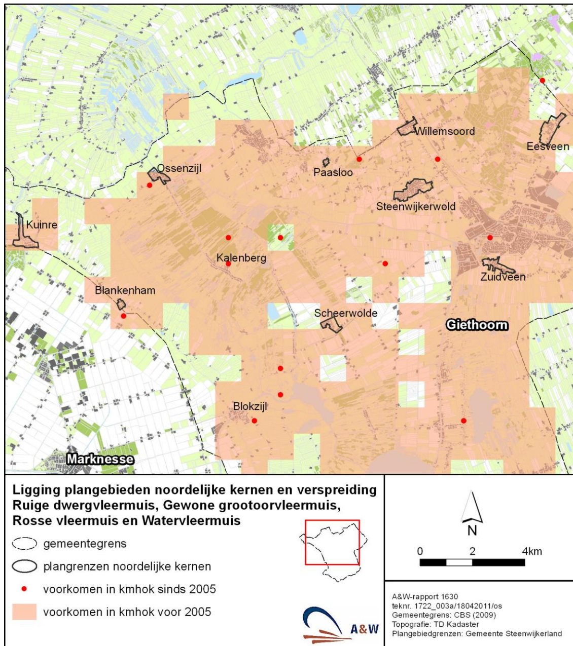
Figuur 3.5 – Verspreiding van boombewonende vleermuizen in de noordelijke kernen.
