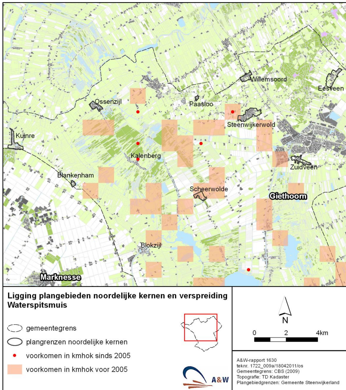
Figuur 3.3 – Verspreiding van de Waterspitsmuis in de noordelijke kernen.
