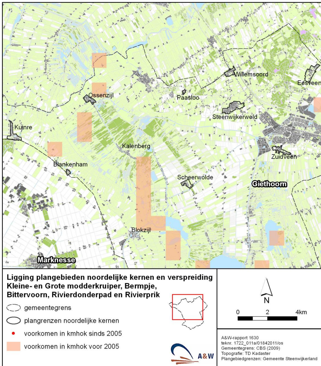
Figuur 3.2 – Verspreiding van vissen in de noordelijke kernen.
