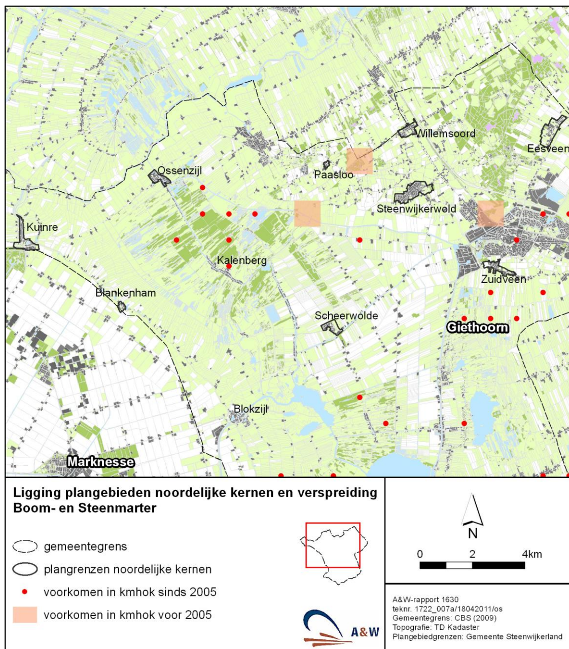
Figuur 3.4 – Verspreiding van Boom- en Steenmarter in de noordelijke kernen.
