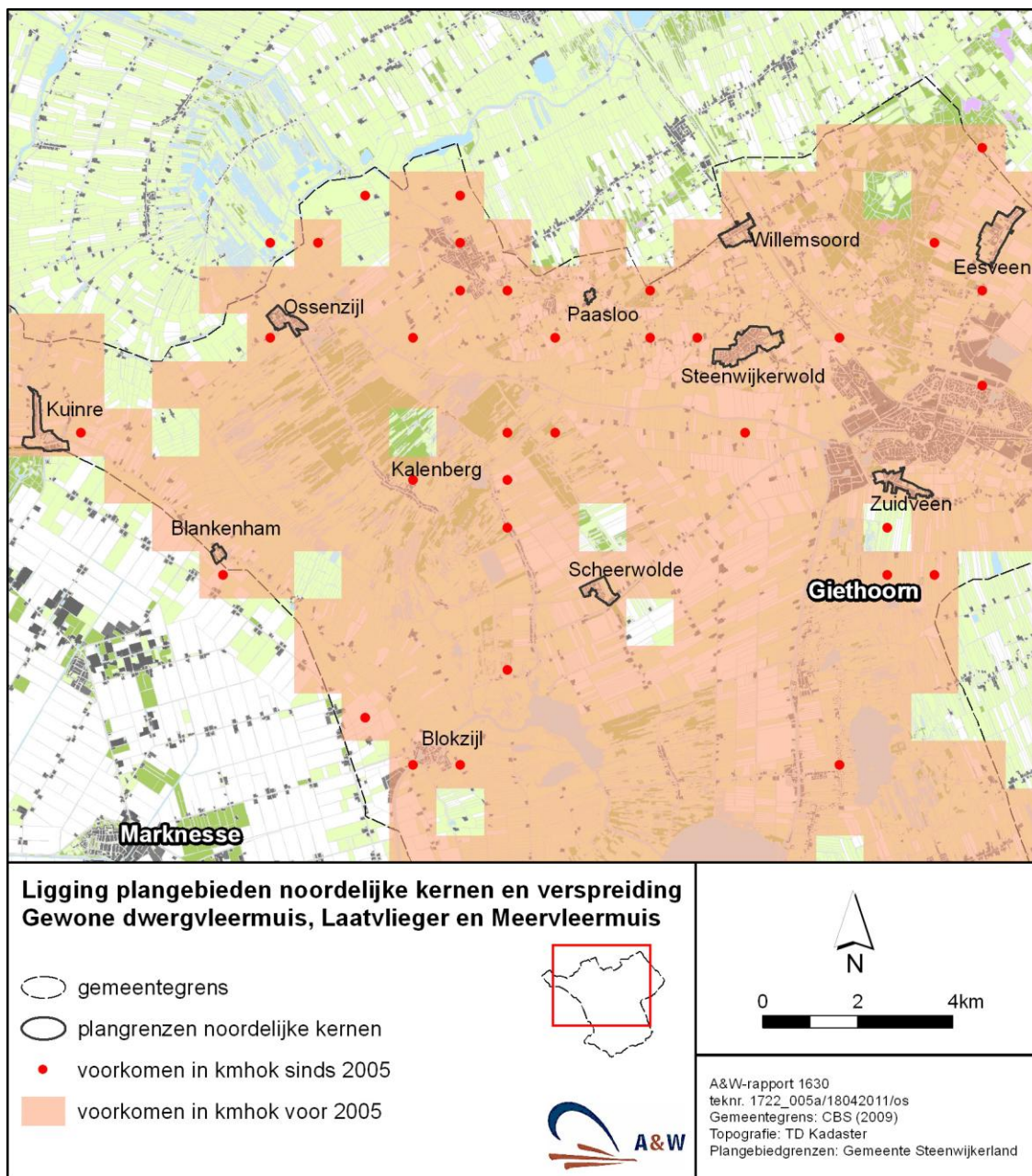
Figuur 3.6 – Verspreiding van huisbewonende vleermuizen in de noordelijke kernen.
